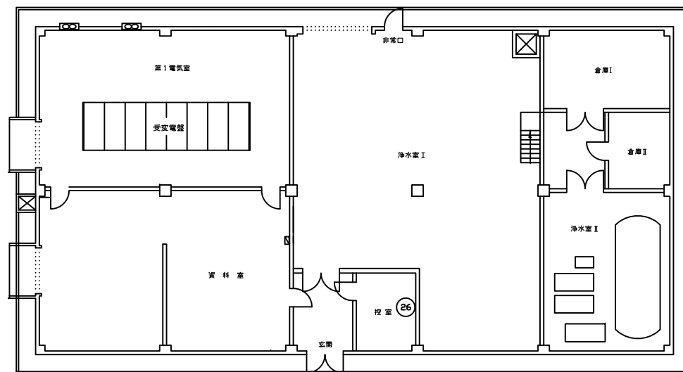
大湊施設 動力棟平面図
