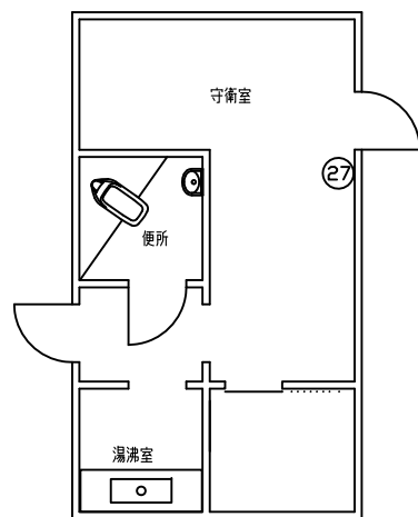
大湊施設 守衛所平面図
