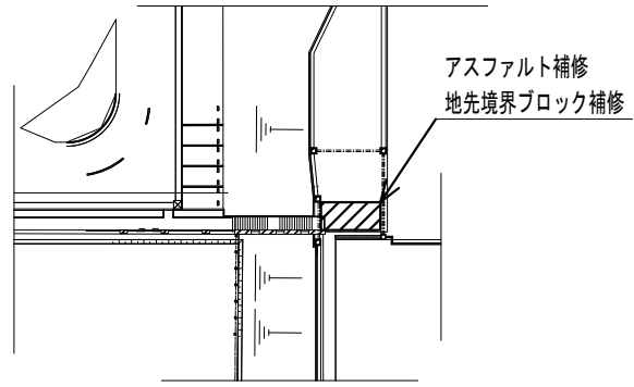
1 犬走り補修 1:1000
