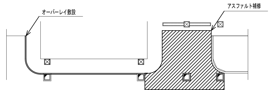
5 試験棟ヤード路床補修 1:200
