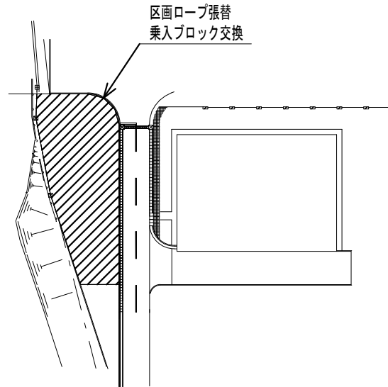
4 砕石駐車場区画ロープ張替 1:1000
