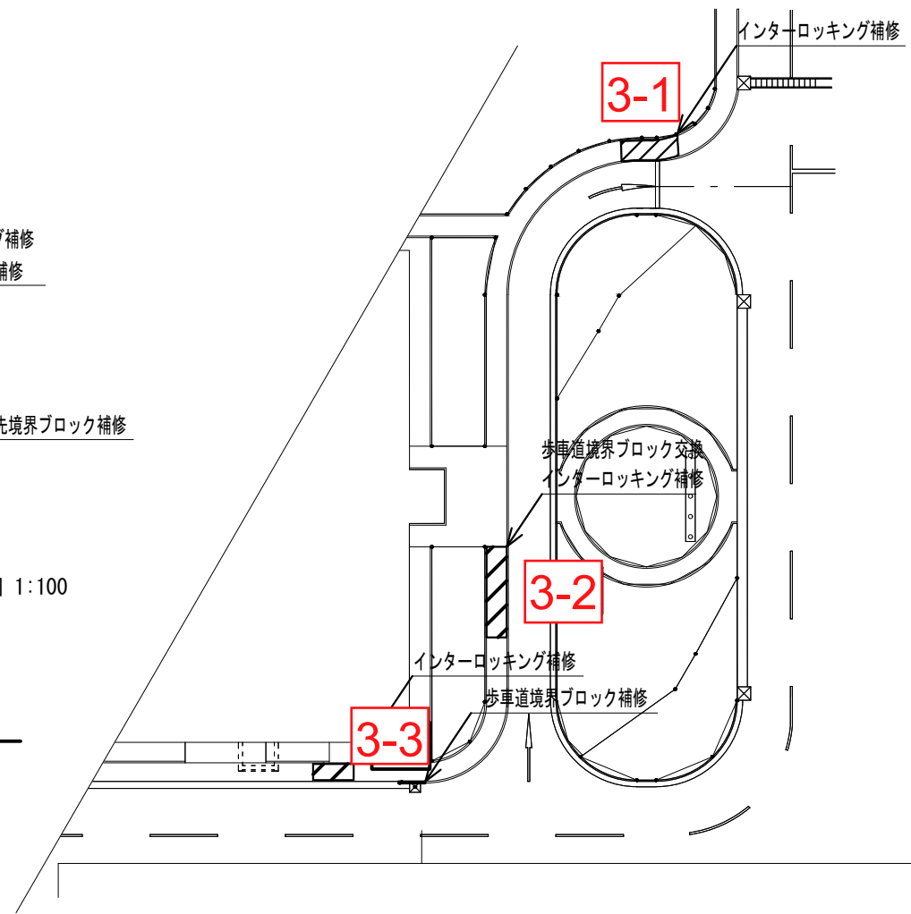
3 石畳補修 1:500
