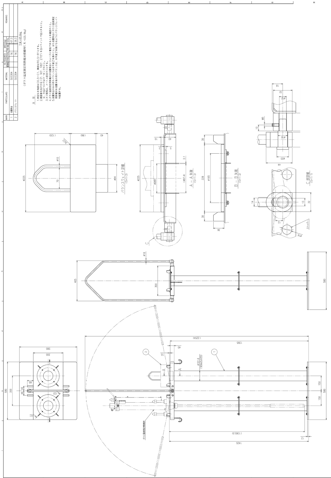
ガラス温度測定用熱電対搬送架台(2本タイプ)概要図
