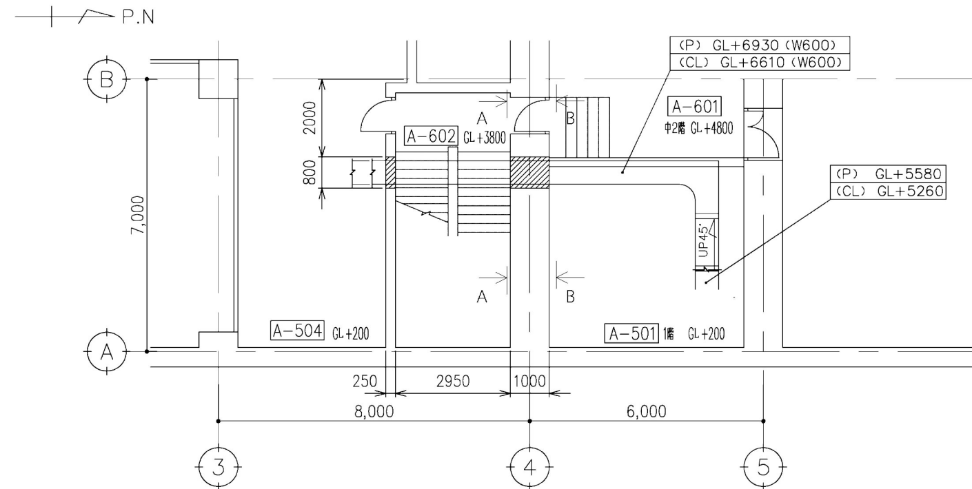
原子炉付属建家M2F A-602付近平面図
