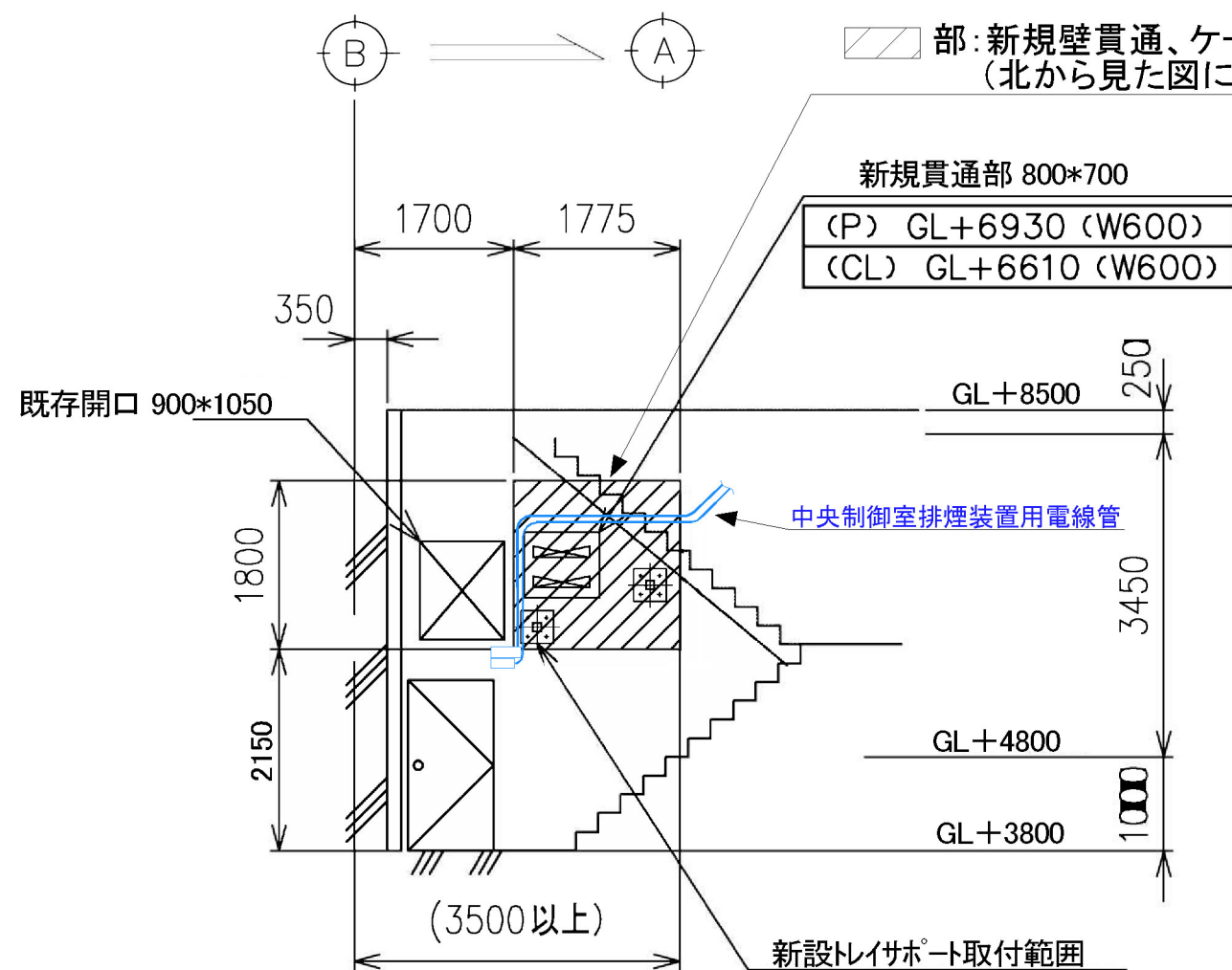
A-A矢視 A-602北壁 (南から見た図)
