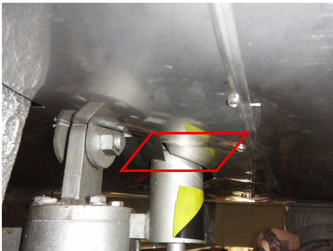
c) 配管サポート No. S-303_PSD-204(A)
