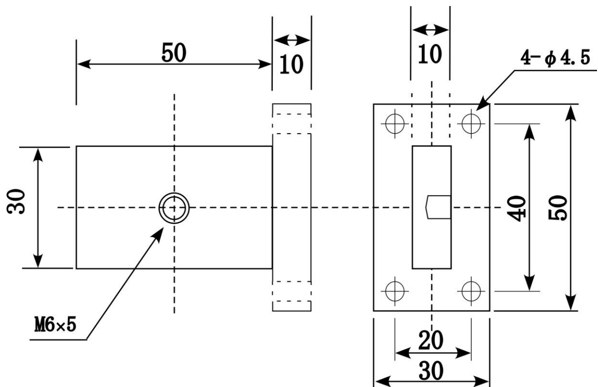
図-1 振動計センサ取付治具の概略図
