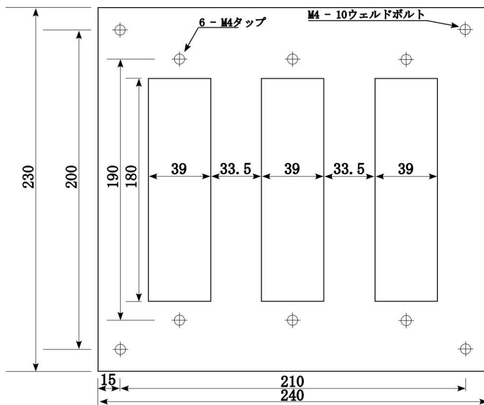
図-2 振動計変換器取付パネルの概略図
