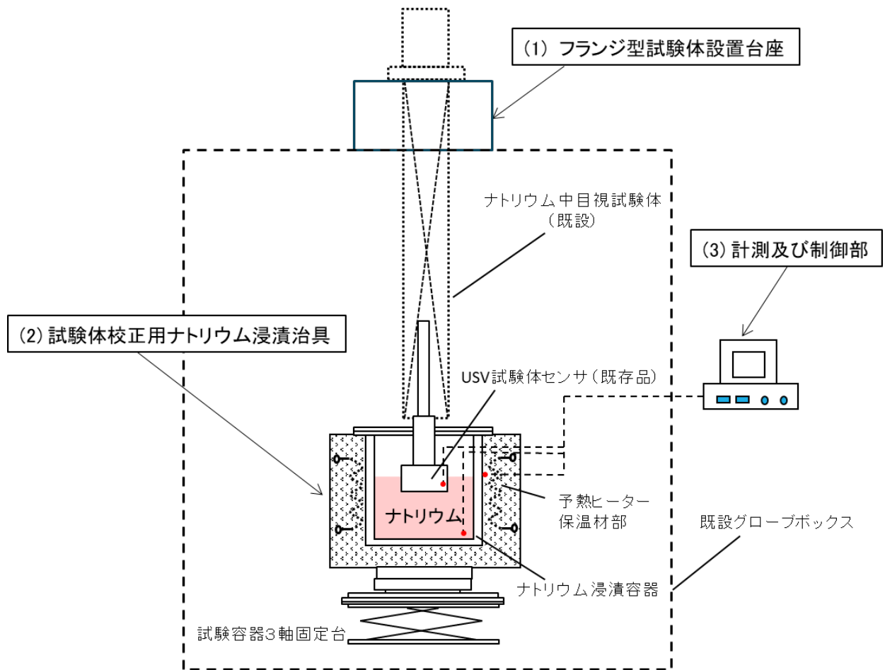
図－1 試験体校正治具の構成概念
