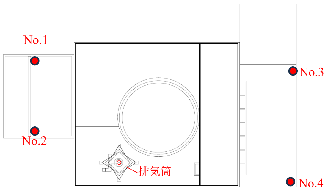
(もんじゅ建屋の屋上図)
