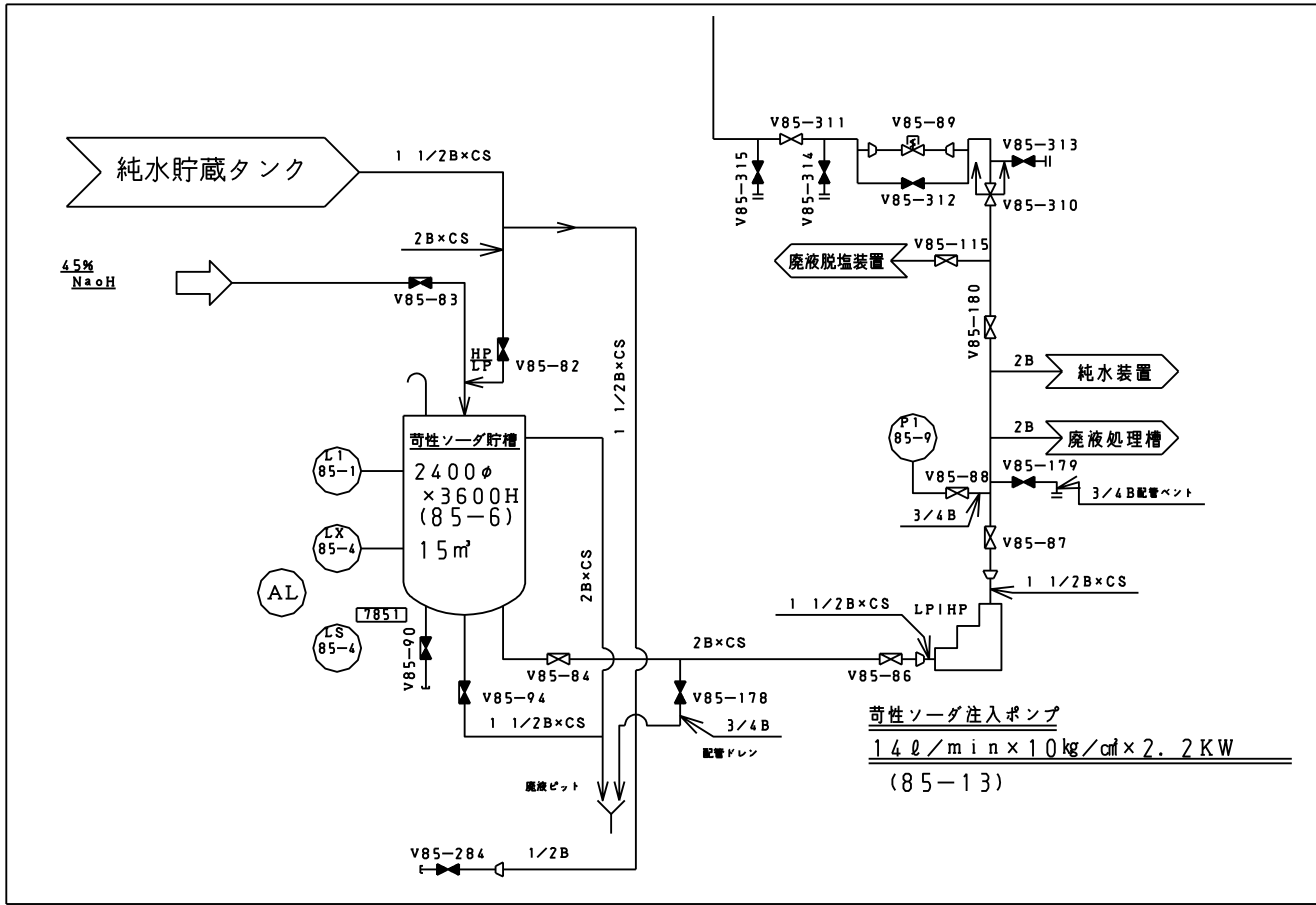
復水脱塩装置系統図 (苛性ソーダ)
