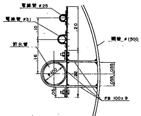
B部詳細断面
