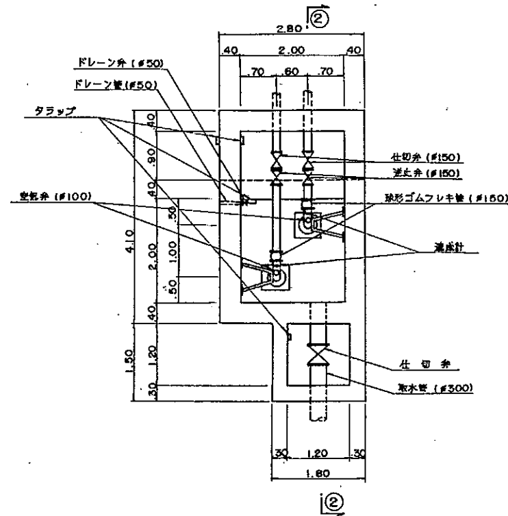
ポンプピット及びバルブピット詳細
