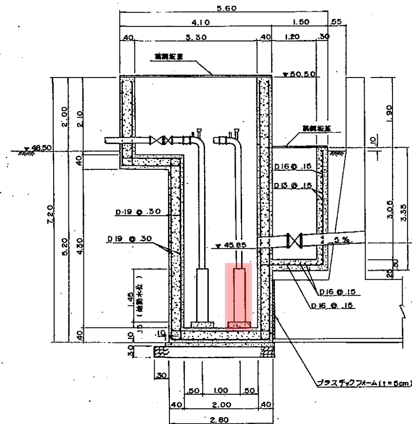
②—② 断面
