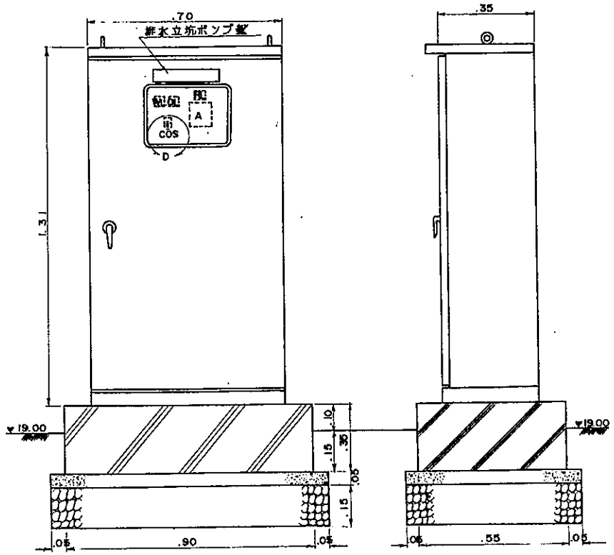
操作盤
