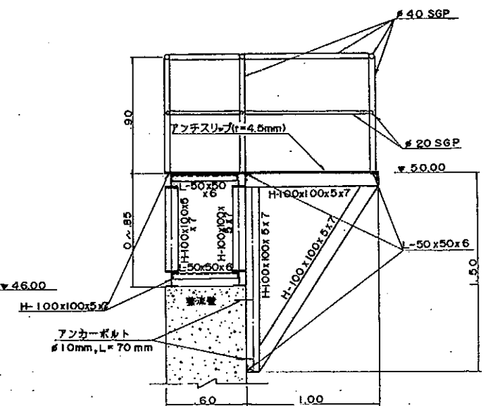
B-B 断面
