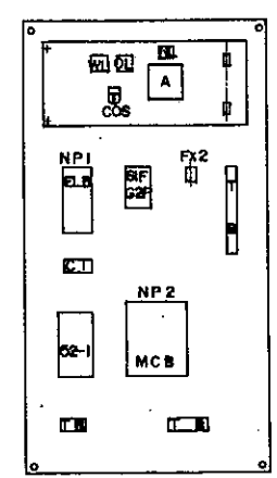
操作盤内配置
