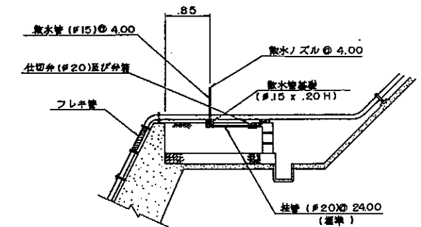
散水管植樹柵部詳細(B)
