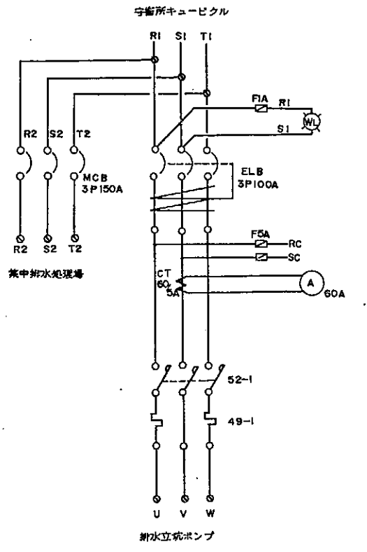
三線結線
