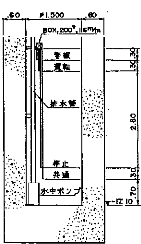
C部詳細
