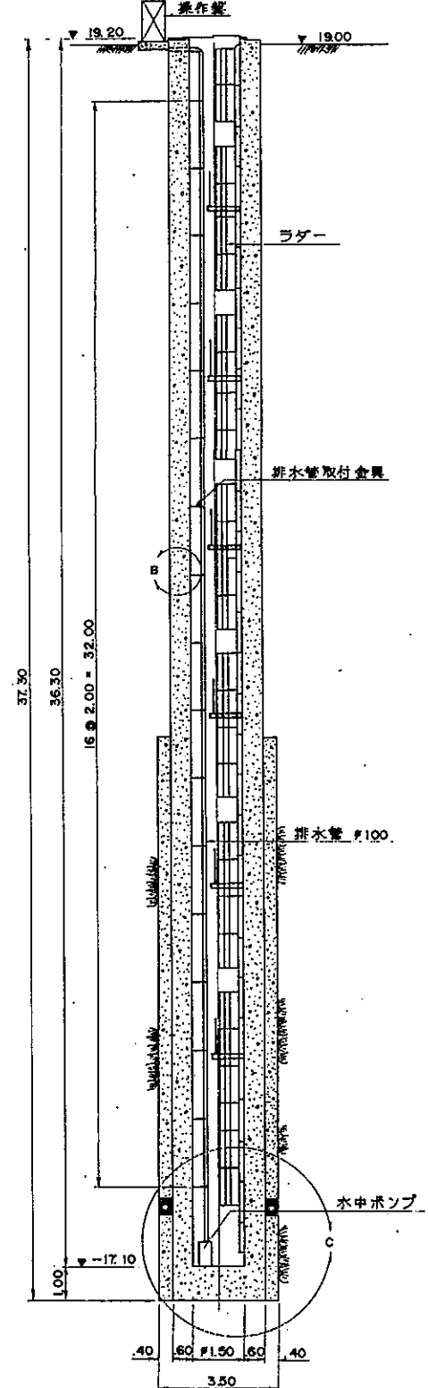
排水立坑断面
