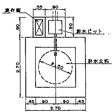
A部詳細
