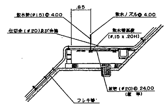
散水管植樹柵部詳細(B)
