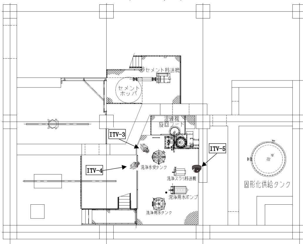
廃棄物処理室 地上 1 階 (GL+2,000~6,500)
