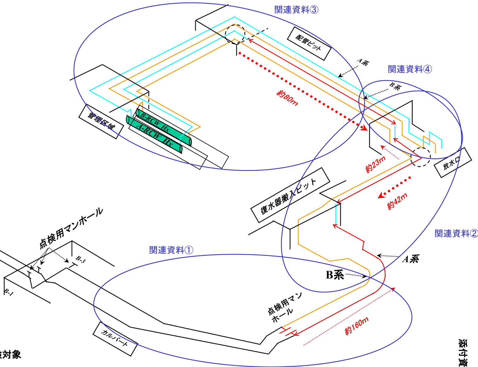
RCWS配管点検範囲図
