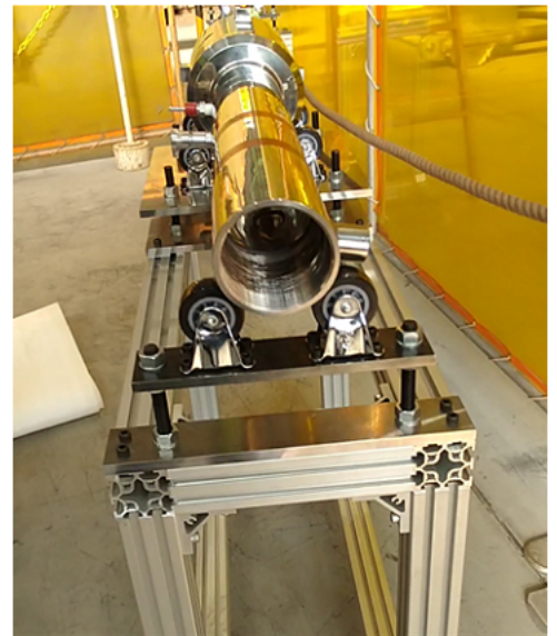
一次蓋吊具用架台 の使用概要
