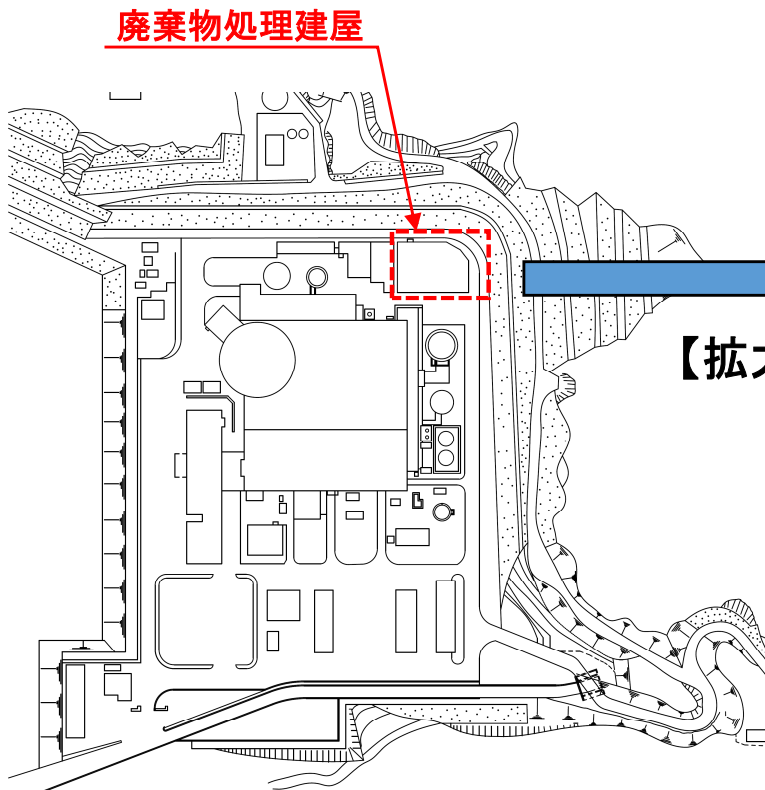
ふげん構内配置図
