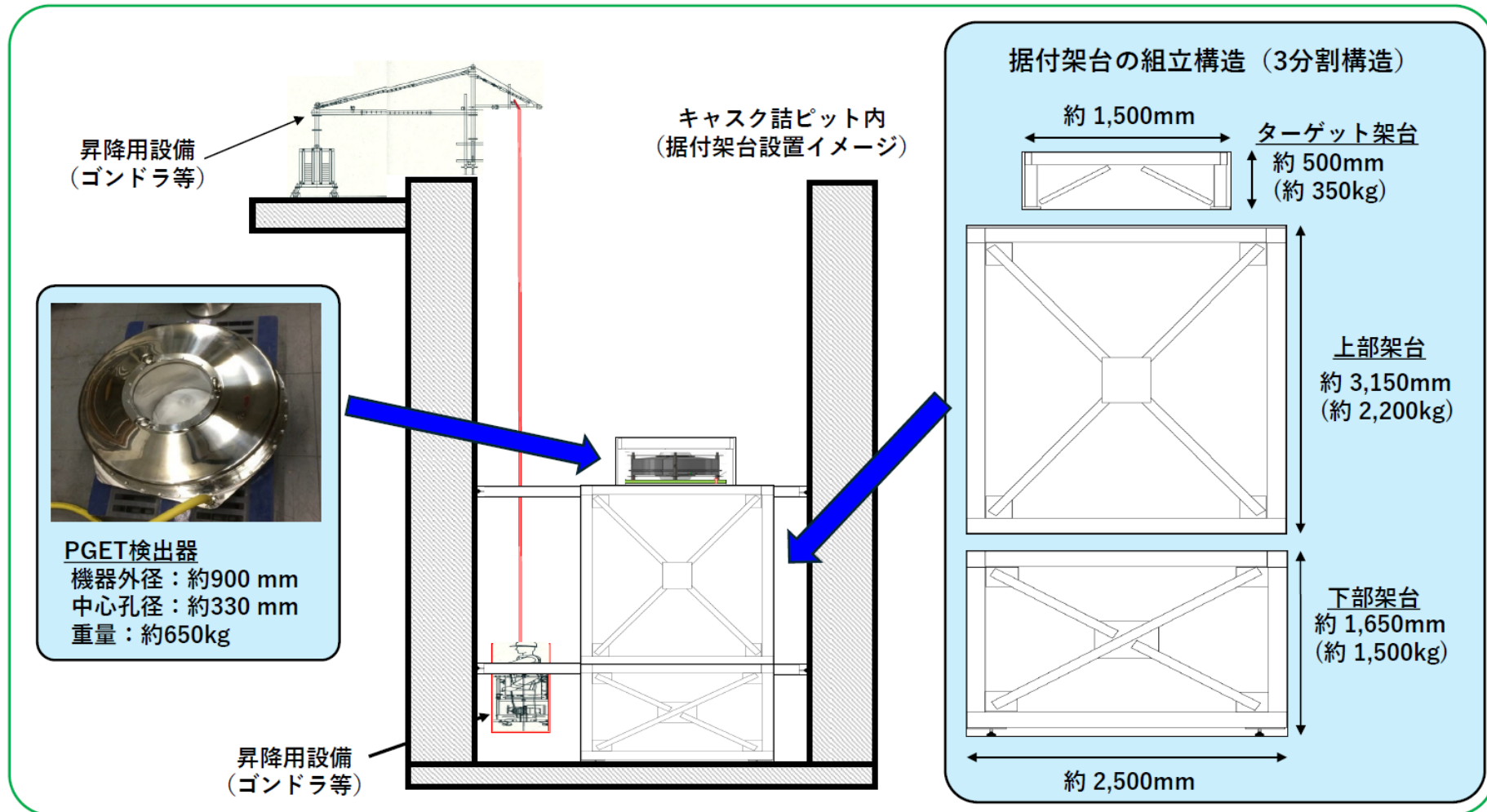
別図3 集合体内部可視化装置及び据付架台の設置作業概要
