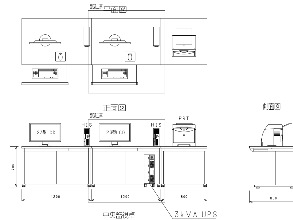
機器外形図
